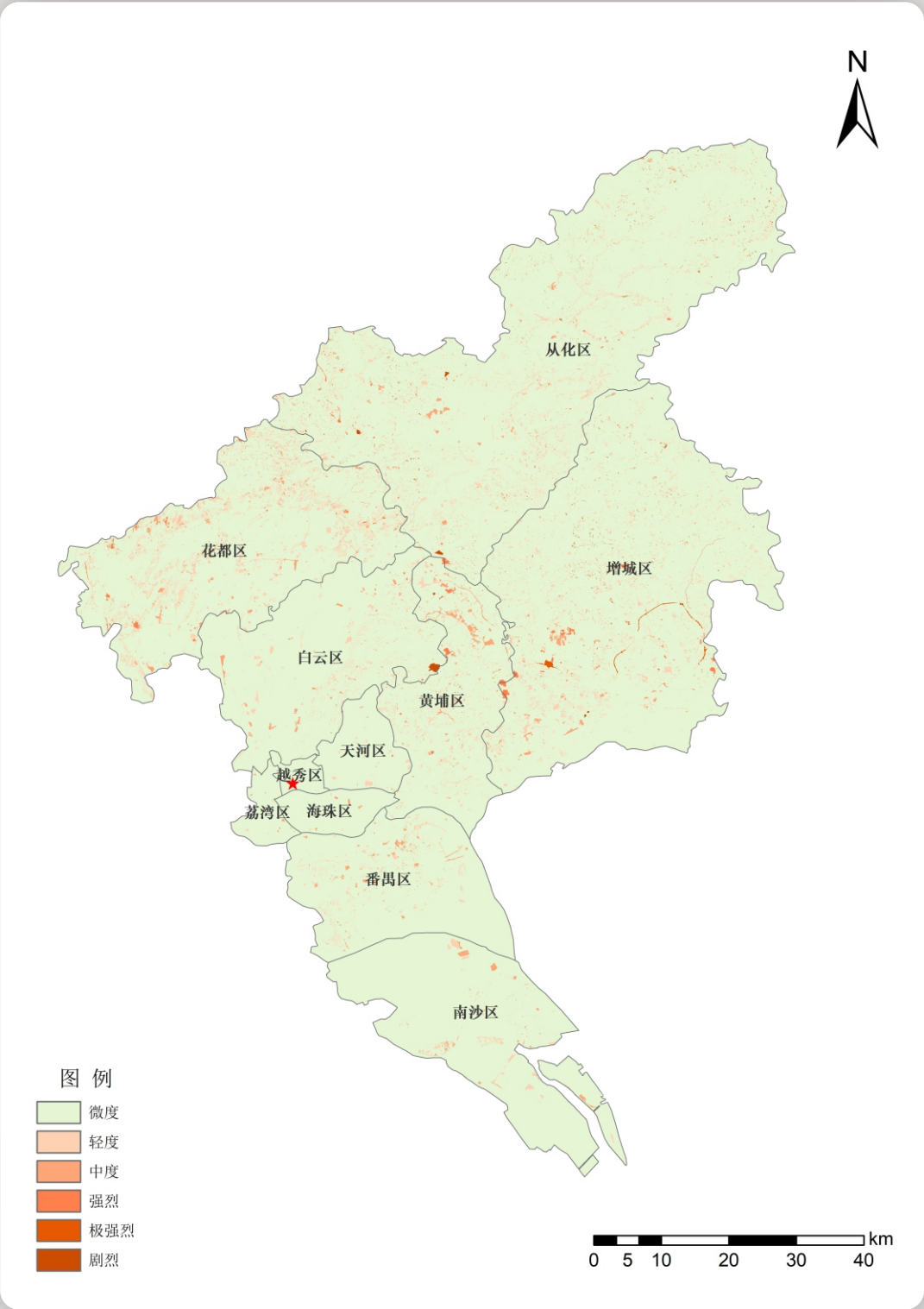
▲图3.2020年广州市土壤侵蚀图
