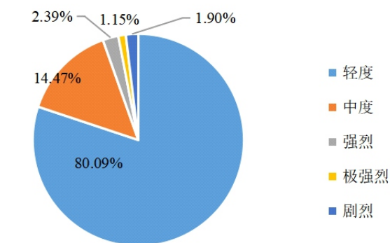
▲图1.广州市各级强度水土流失面积比例图
