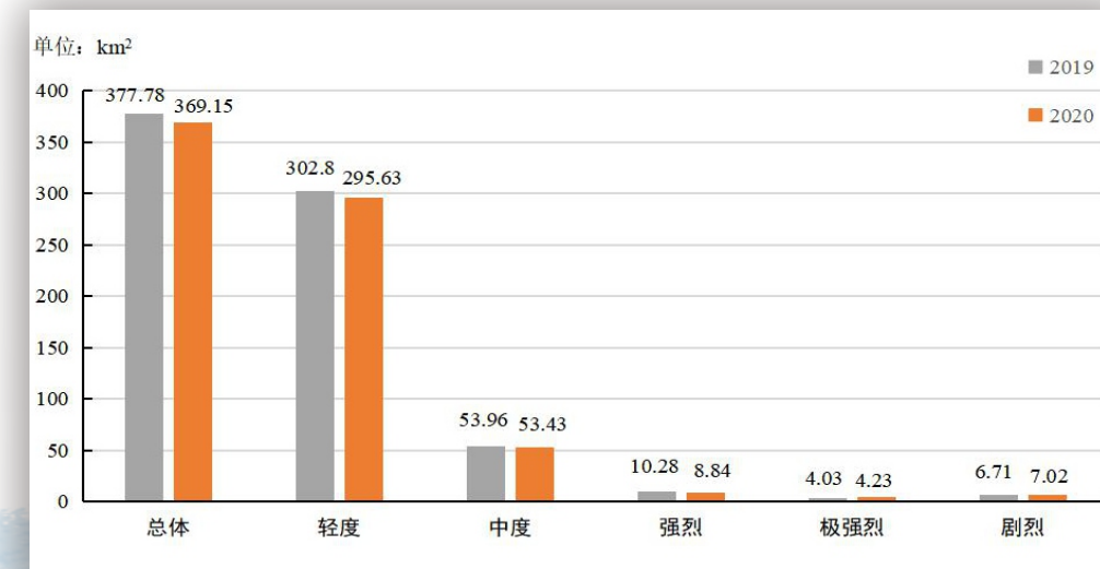
▲图2.广州市水土流失面积变化图
